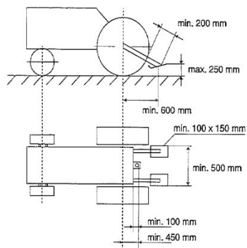
Figuur 14-1: constructie/maatvoering steigerbegrenzer
